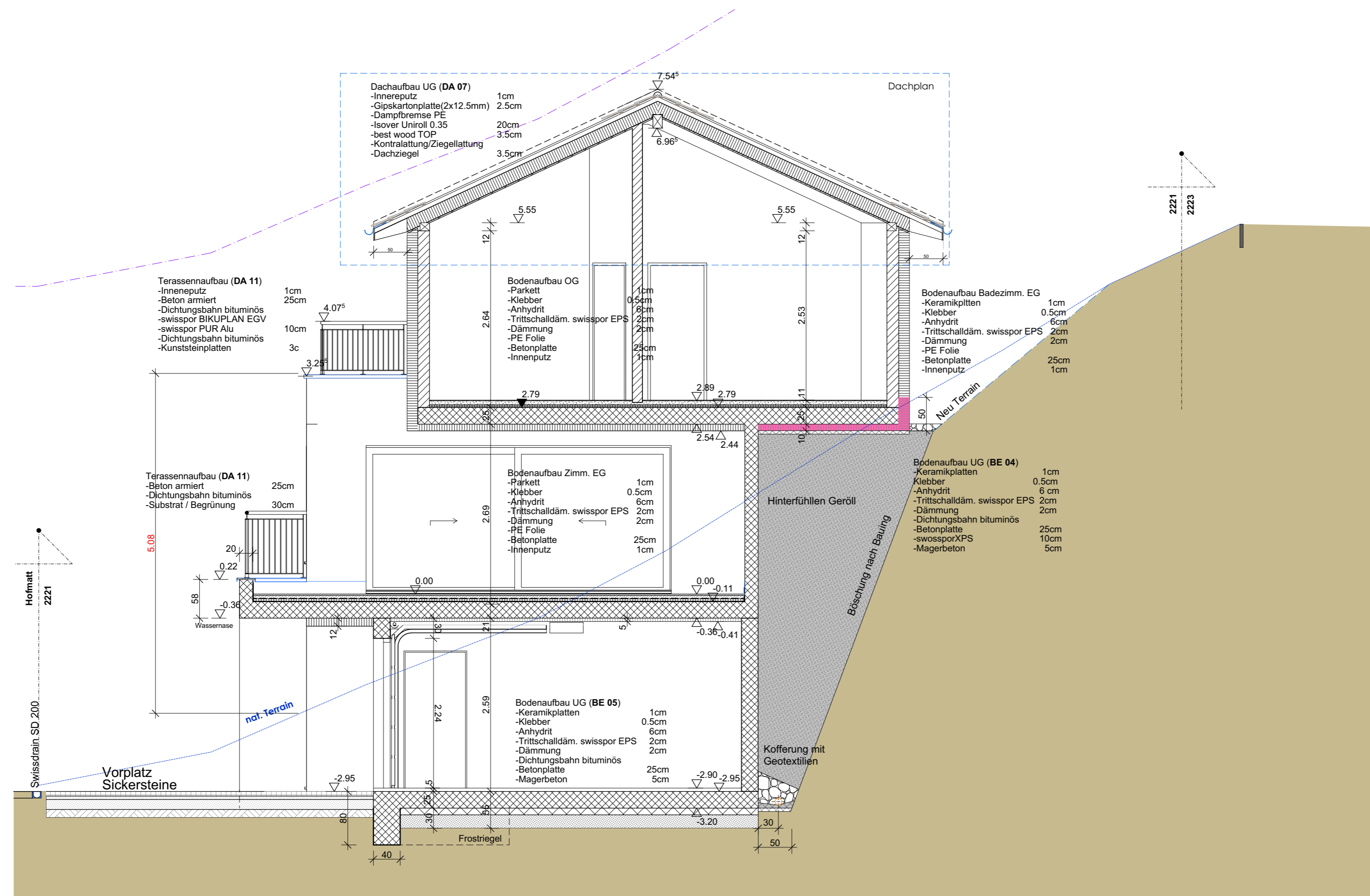
SCHNITT C_C
